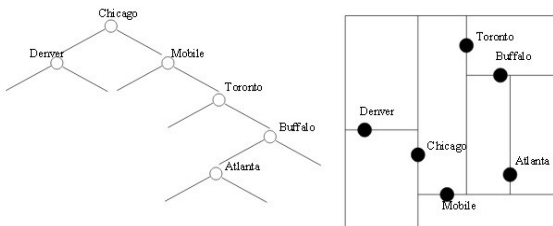
Obr. 3: Příklad kd stromu pro k=2 [6].
